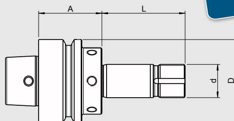
Zeichnung und Abbildung zeigen Schleifscheibenaufnahme für HSK-F50 ISOG Drawing and picture show grinding wheel adapter for HSK-F50 ISOG
