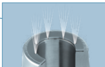
Optimierte Kühlmittelbohrung mit KSS-Austritt durch Schlitze Cool Flash System von HAIMER
